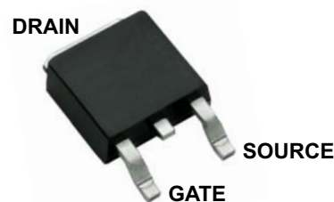
TO-252 (D-PAK) (K4)
