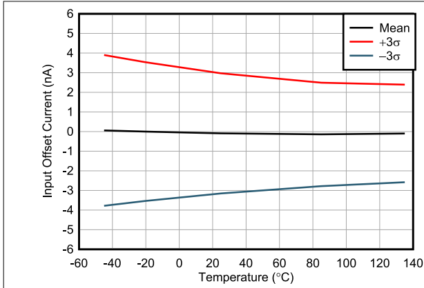
图 7-19. 输入失调电流与温度间的关系
