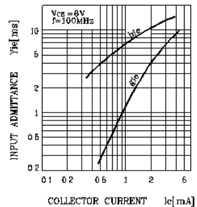
■ Fig. 6 I_C-Y_{ie}
