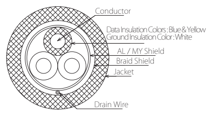
CC-Link Cable
