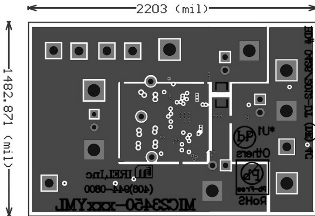
Bottom Layer
