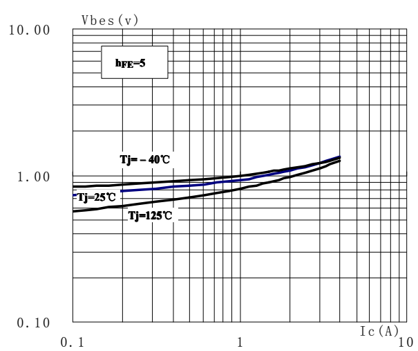
V_{besat} - I_c
