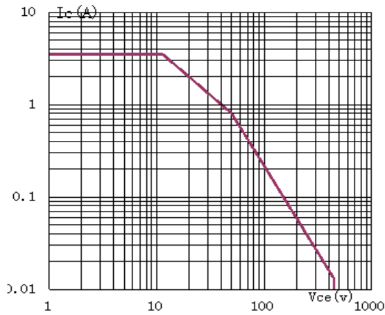
SOA (DC)
