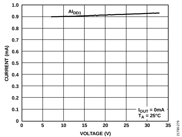
Figure 71. ALDD1 Current vs AVDD1 Supply
