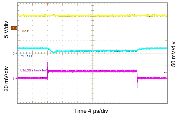
图 87. 3.3 V_{SLSDO} Load Transient, 0 to 10 mA
