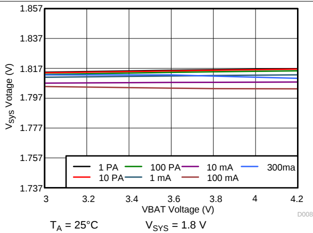
图 58. 1.8 V_{SYS} Line Regulation
