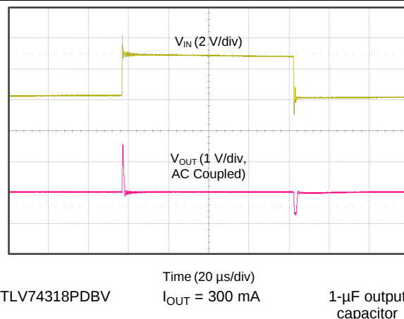
图 24. Line Transient
