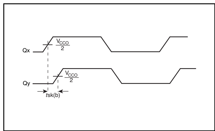
Output Skew
