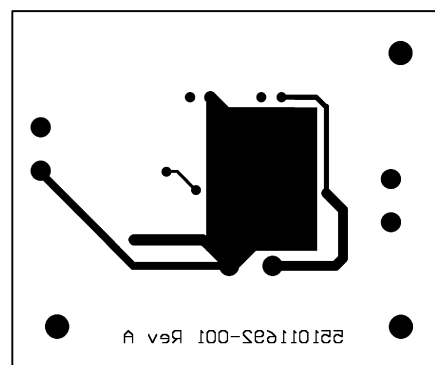
Bottom Layer
