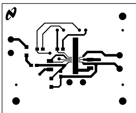
Top Layer
