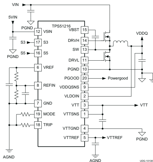
应用示意图
