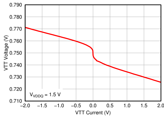
图 7-18. VTT Load Regulation
