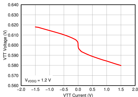
图 7-20. VTT Load Regulation
