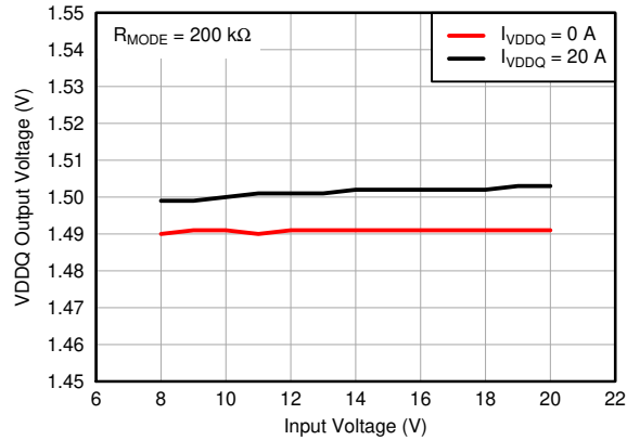
图 7-14. Line Regulation
