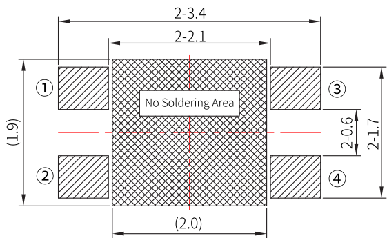
RECOMMEDED P.C.B LAYOUT 安装尺寸图
