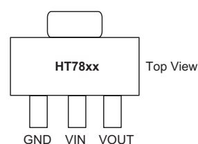
SOT89
