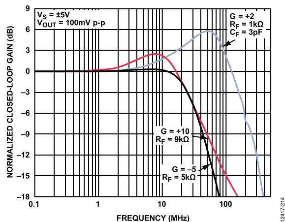
图16. 不同增益下的小信号频率响应 ( V_S = \pm 5\text{ V} , 见图51和图52中的测试电路)
