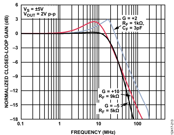
图18. 不同增益下的大信号频率响应 ( V_S = \pm 5\text{ V} , 见图51和图52中的测试电路)
