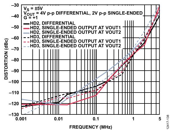
图38. 谐波失真与频率的关系
