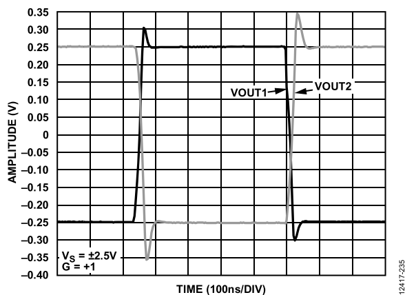
图36. 大信号阶跃响应(单端输出), V_S = \pm 2.5\text{ V}
