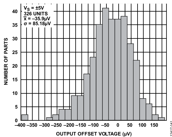
图39. 差分输出失调电压
