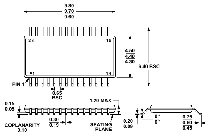
图74. 28引脚超薄紧缩小型封装[TSSOP] (RU-28) 图示尺寸单位: mm
