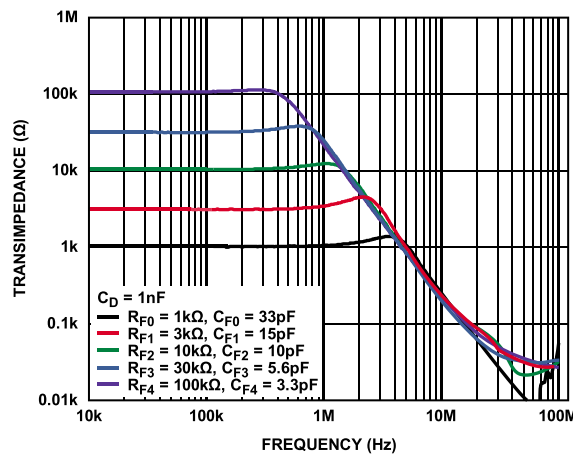
图64. 跨阻与频率的关系, C_D = 1 nF
