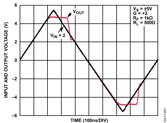
图45. 输出过驱恢复(仅M1)
