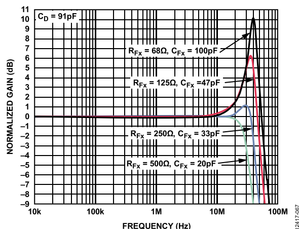
图68. 降低 R_F 时的归一化频率响应(见图67)
