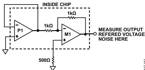
图54. P1和M1的折合到输出端电压噪声
