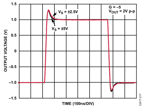
图20. 不同电源下的大信号阶跃响应, G = -5
