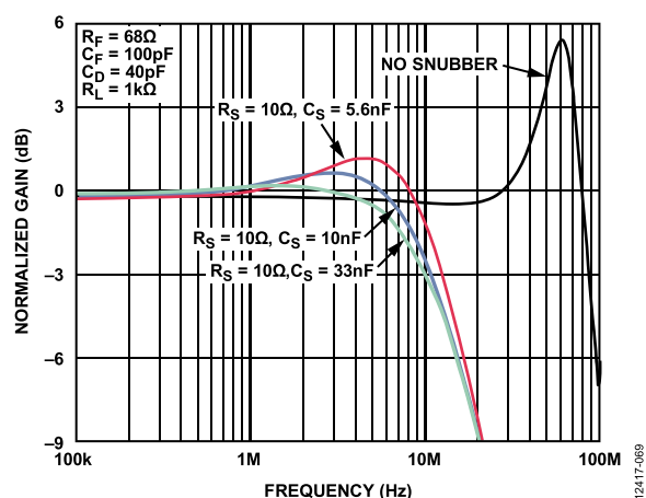
图70. 缓冲器电路对跨阻频率响应的影响(见图69)
