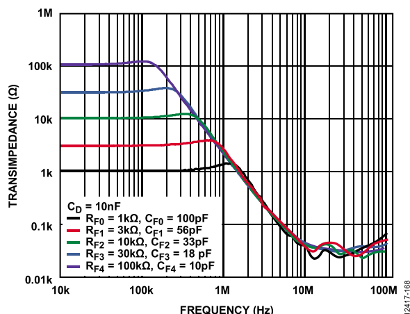
图65. 跨阻与频率的关系, C_D = 10 \text{ nF}
