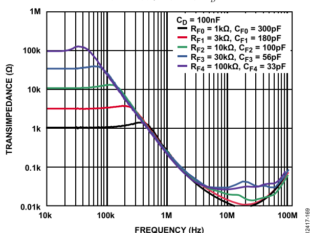
图66. 跨阻与频率的关系, C_D = 100 \text{ nF}
