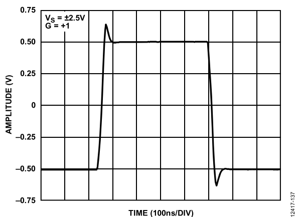
图37. 大信号阶跃响应(差分输出), V_S = \pm 2.5\text{ V}
