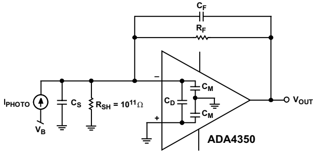
图59. ADA4350的跨阻放大器模型
