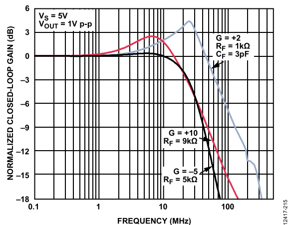
图19. 不同增益下的大信号频率响应 ( V_S = 5\text{ V} , 见图51和图52中的测试电路)
