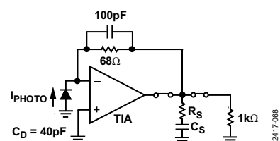
图69. 增加缓冲器电路以减轻峰化
