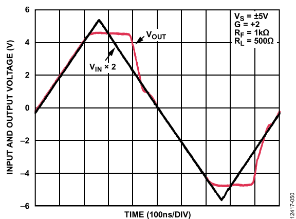
图44. 输出过驱恢复(仅P1)
