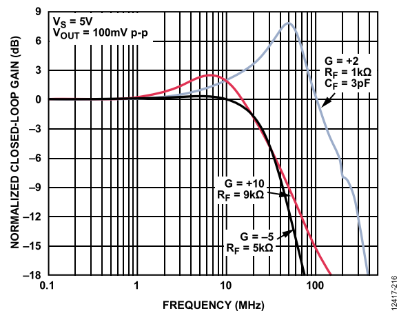
图17. 不同增益下的小信号频率响应 ( V_S = 5\text{ V} , 见图51和图52中的测试电路)
