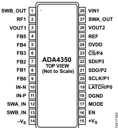
图6. 引脚配置
