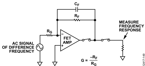
图52. FET输入放大器的频率响应，反相增益配置
