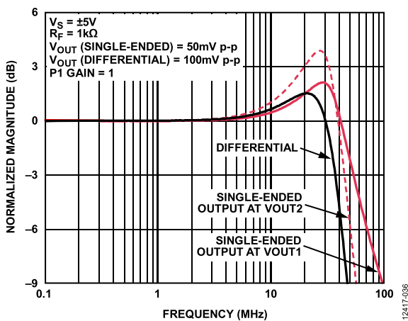
图32. 小信号频率响应, V_S = \pm 5\text{ V}
