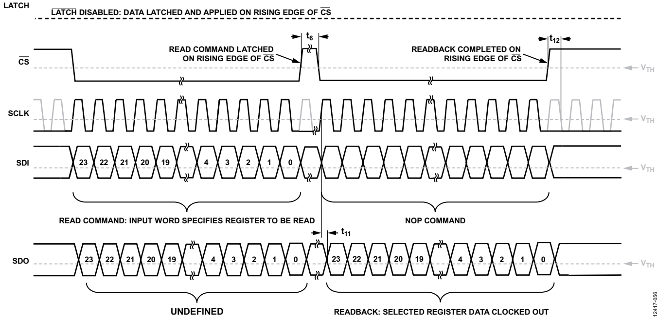
图3. 读操作
