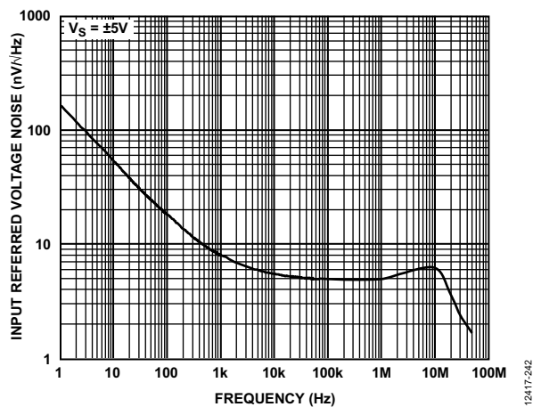
图47. 折合到输入端电压噪声与频率的关系 (仅P1, 见图53中的测试电路)
