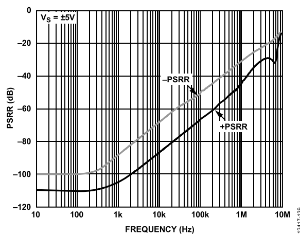
图46. PSRR与频率的关系(仅P1)
