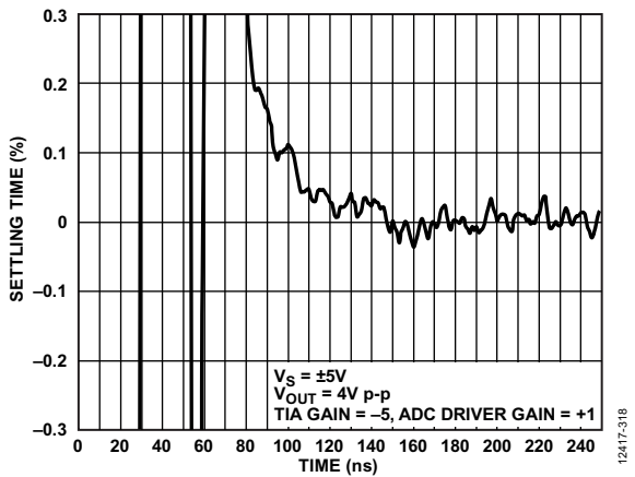
图14. 0.1%建立时间(见图50中的测试电路)
