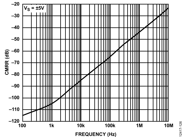
图27. CMRR与频率的关系
