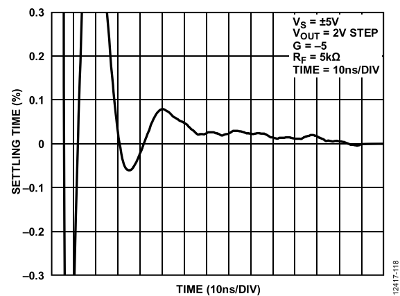
图21. 0.1%建立时间
