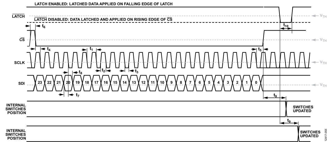
图2. 写操作
