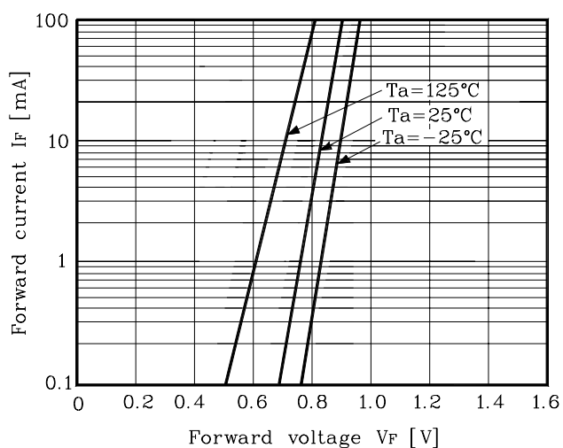
Fig. 3 I_F - V_F
