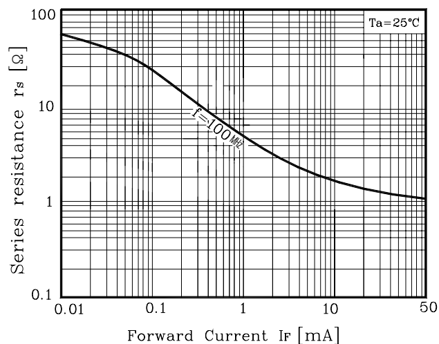
Fig. 1 r_s - I_F
