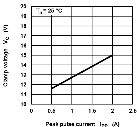
Fig. 8.1 V_C - I_{PP}
