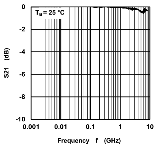
Fig. 9.1 S_{21} - f
