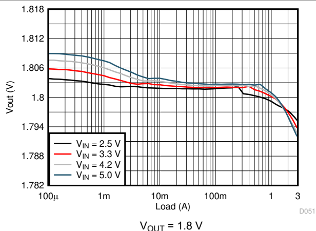
图 9-16. Load Regulation
