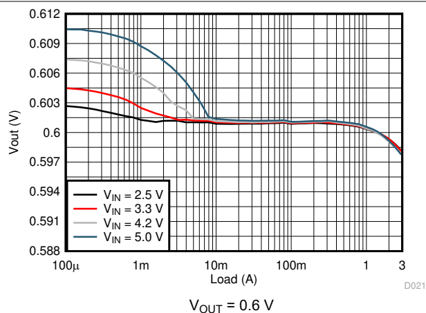
图 9-4. Load Regulation
