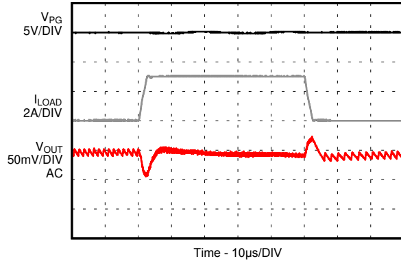
图 9-33. Load Transient
