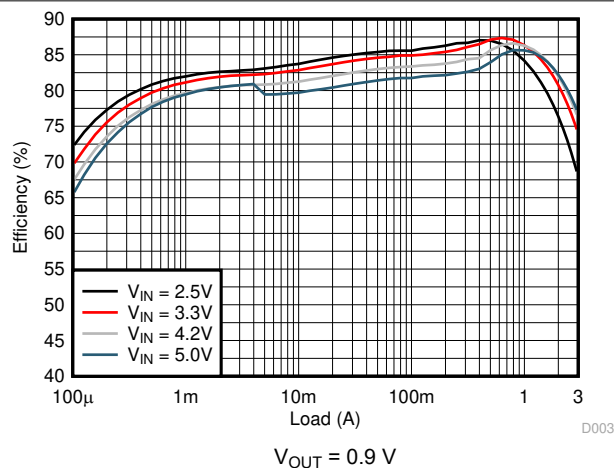
图 9-7. Efficiency
