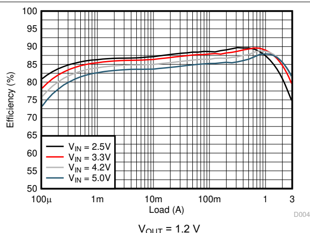
图 9-11. Efficiency
