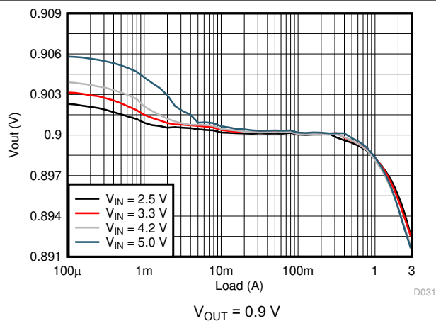
图 9-8. Load Regulation
