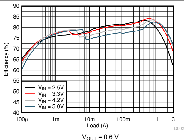
图 9-3. Efficiency
