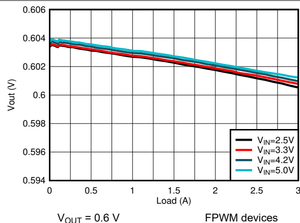
图 9-6. Load Regulation
