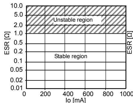
Fig. 28 BA3259HFP ESR
