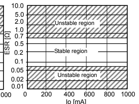
Fig. 29 BA30E00WHFP ESR
