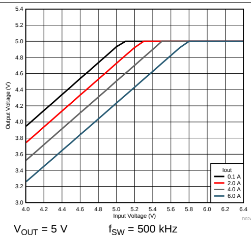
图 41. Voltage Dropout
