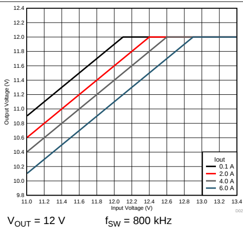
图 43. Voltage Dropout
