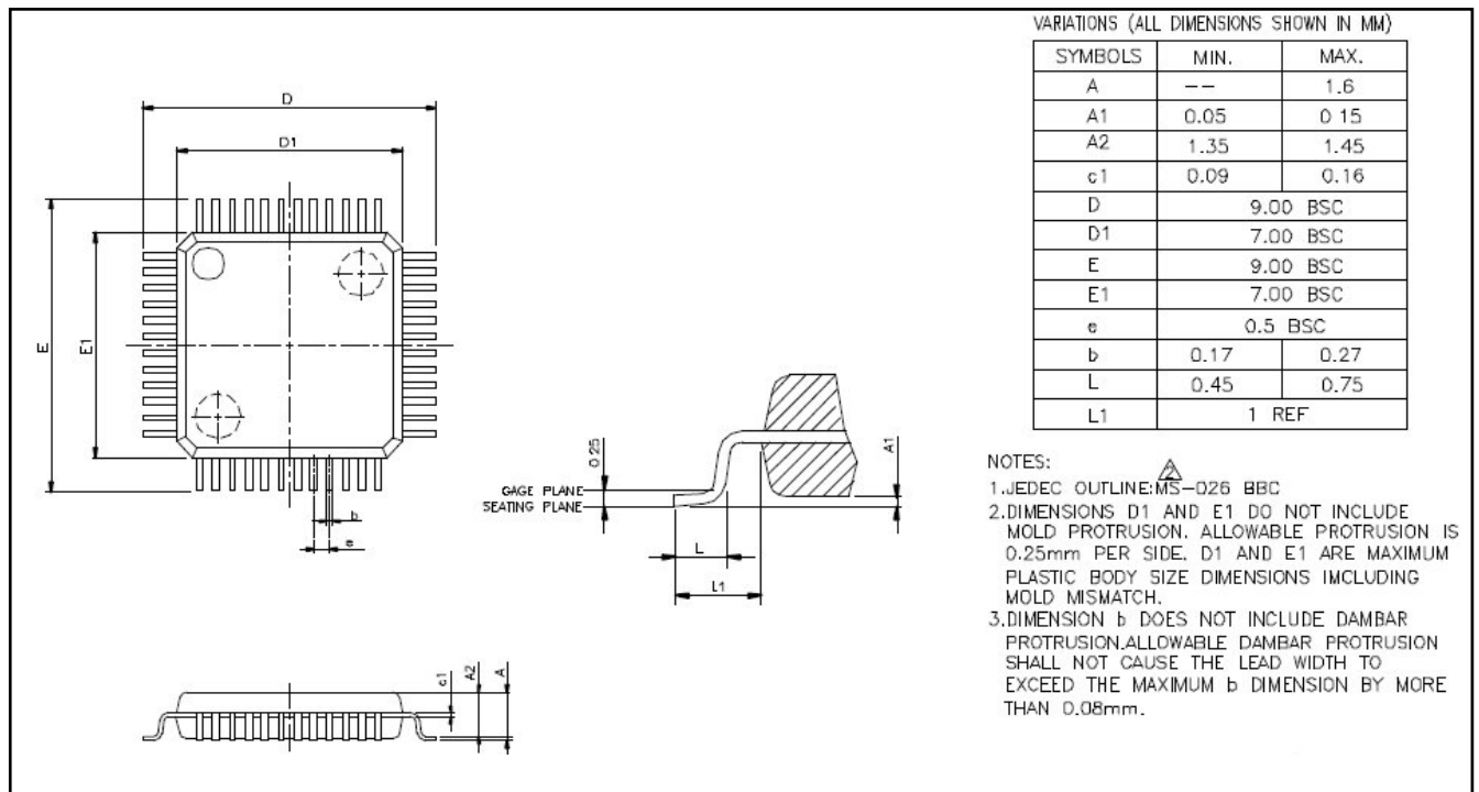
MG84FL54BD (LQFP-48)
