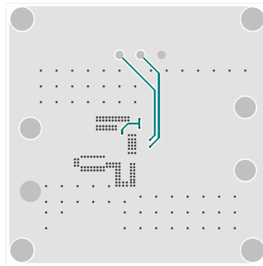
Figure 4—Bottom Layer
