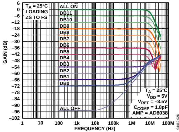
图20. 基准乘法带宽与频率和代码的关系
