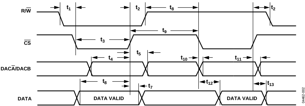
图2. 时序图
