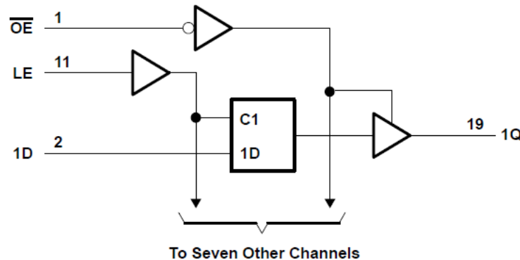
功能方框图
