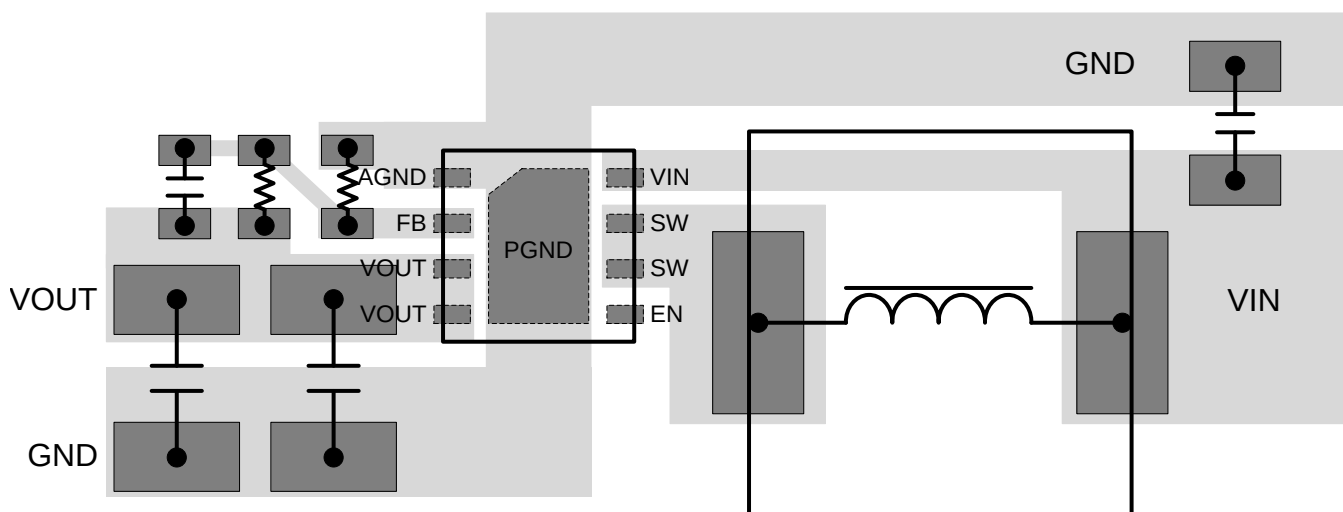
图 18. Layout Example
