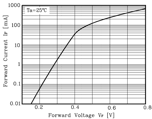
Fig. 1 I_F - V_F
