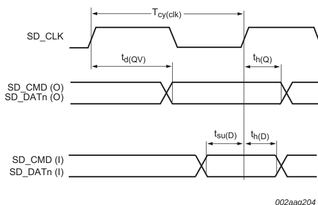
Fig 27. SD/MMC timing
