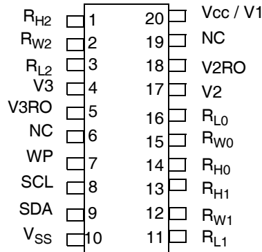
20 Pin TSSOP
