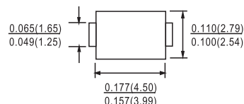
DO-214AC(SMA)
