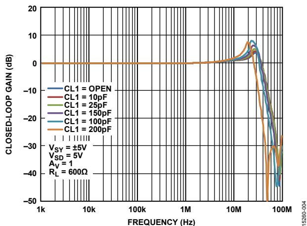
图4. 不同容性负载下的频率响应, V_{SY} = \pm 5V
