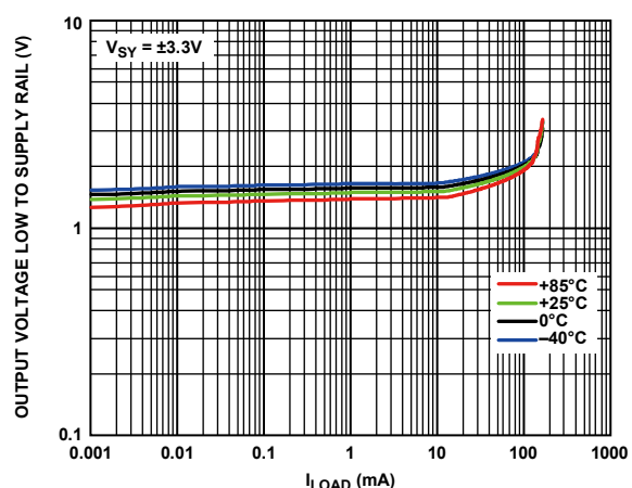
图26. 输出低电压( V_{OL} )至供电轨与负载电流( I_{LOAD} )的关系, V_{SY} = \pm 3.3\text{ V}
