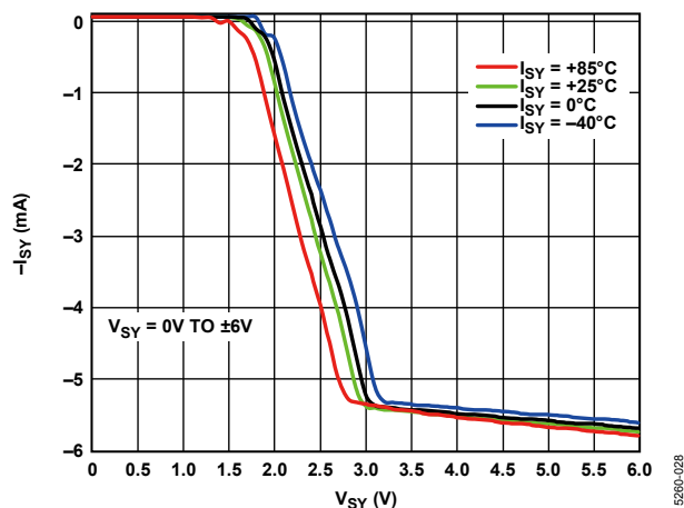
图28. 电源电流( -I_{SY} )与电源电压( V_{SY} )的关系
