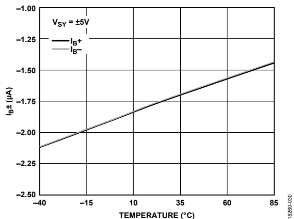
图30. 输入偏置电流( I_{B\pm} )与温度的关系, V_{SY} = \pm 5\text{ V}
