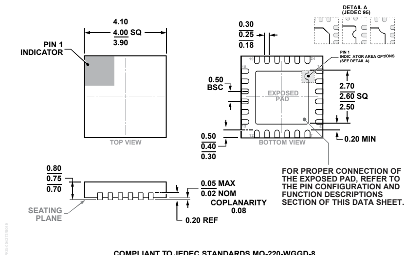
图49. 24引脚引线框芯片级封装[LFCSP]
