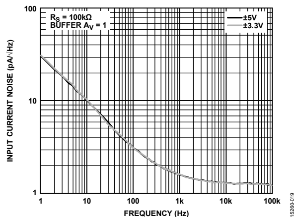
图19. 输入电流噪声与频率的关系
