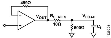
图43. 驱动容性负载的原理图
