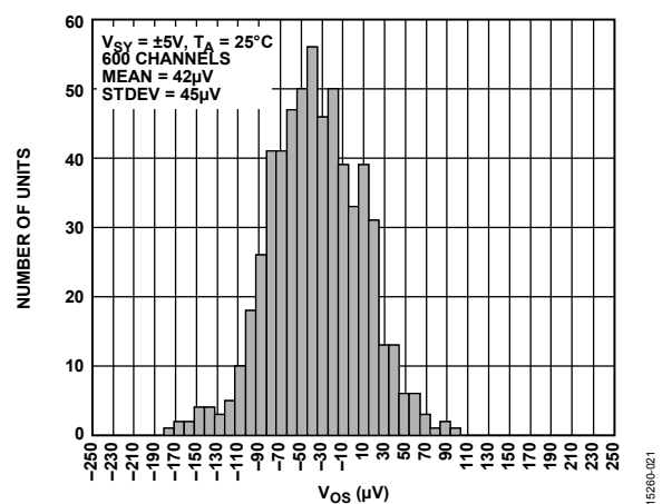
图21. 输入失调电压( V_{OS} )分布, V_{SY} = \pm 5V
