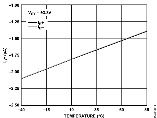
图31. 输入偏置电流( I_{B\pm} )与温度的关系, V_{SY} = \pm 3.3\text{ V}
