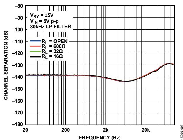
图8. 通道隔离与频率的关系, V_{SY} = \pm 5V
