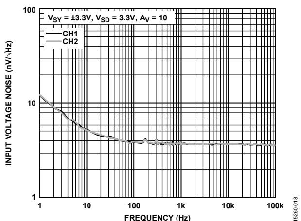
图18. 输入电压噪声与频率的关系, V_{SY} = \pm 3.3V
