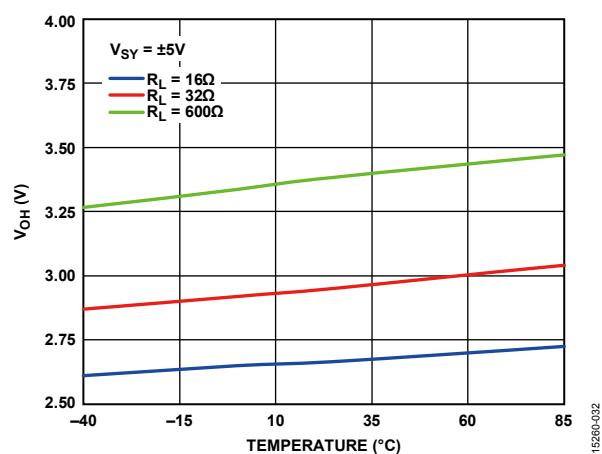
图32. 输出高电压( V_{OH} )与温度的关系, V_{SY} = \pm 5\text{ V}
