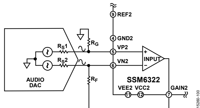
图40. 无共模控制的共模电路
