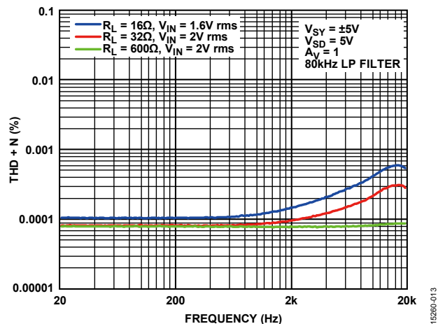
图13. THD + N与频率的关系, V_{SY} = \pm 5V
