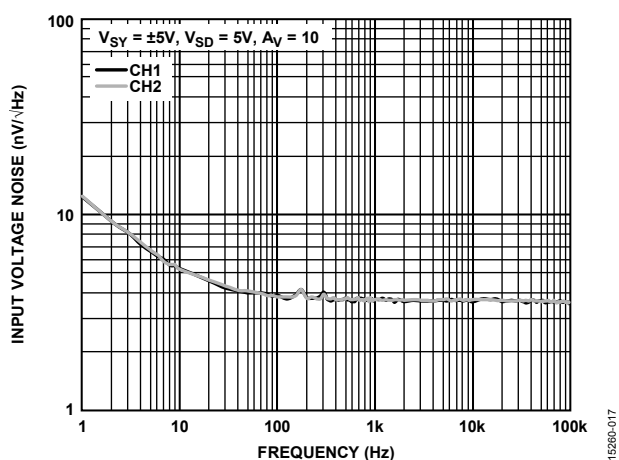
图17. 输入电压噪声与频率的关系, V_{SY} = \pm 5V
