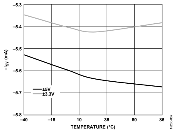
图37. 电源电流( -I_{SY} )与温度的关系
