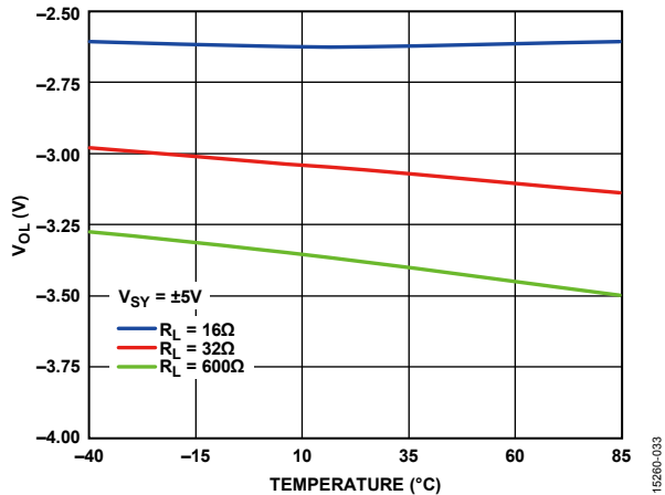
图33. 输出低电压( V_{OL} )与温度的关系, V_{SY} = \pm 5\text{ V}
