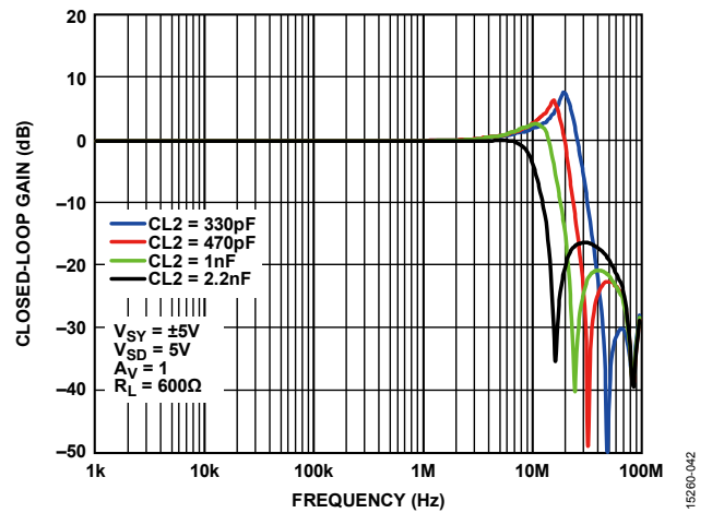
图44. 驱动容性负载的频率响应， V_{SY} = \pm 5\text{ V}
