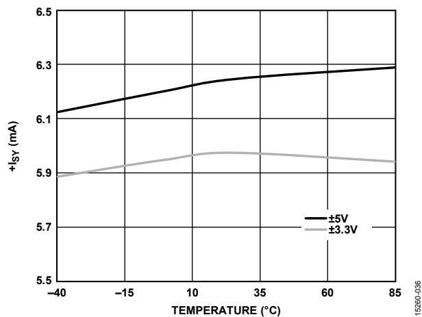
图36. 电源电流( +I_{SY} )与温度的关系
