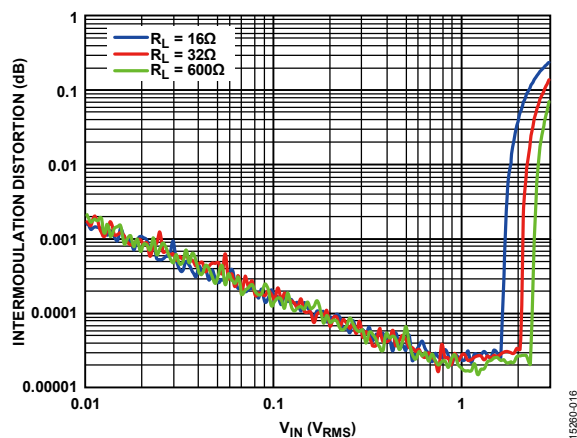
图16. CCIF与输入电压( V_{IN} )的关系, V_{SY} = \pm 5V
