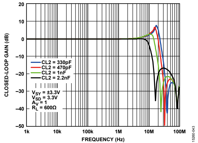
图45. 驱动容性负载的频率响应， V_{SY} = \pm 3.3\text{ V}
