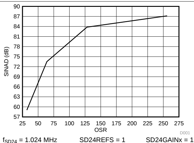
Figure 5-8. SINAD vs OSR
