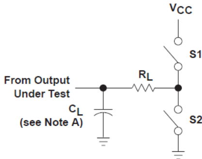
图 6-1. Load Circuit
