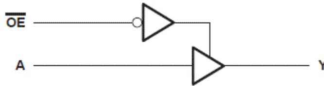
功能方框图
