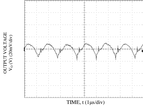
Vo=1.2V, Io = Io,max, Vin=12V
