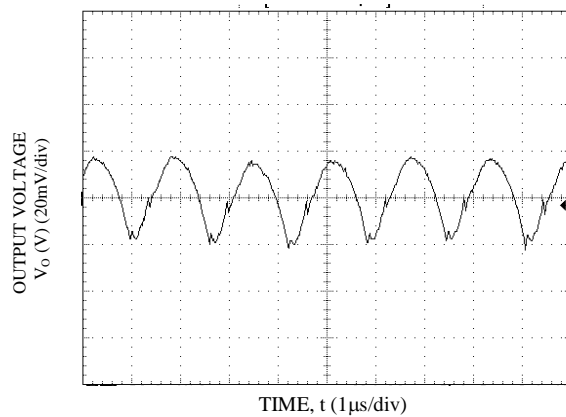
Vo=2.5V, Io = Io,max, Vin=12V
