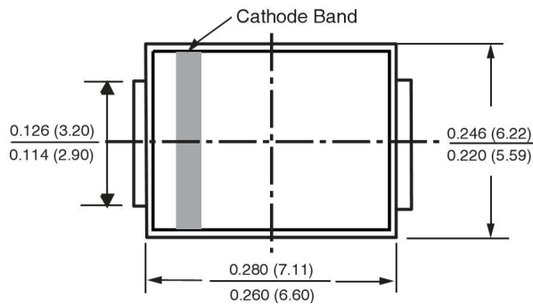
DO-214AB(SMC)
