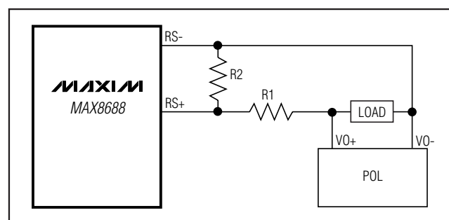
Figure 16. VOUT_SCALE_LOOP
