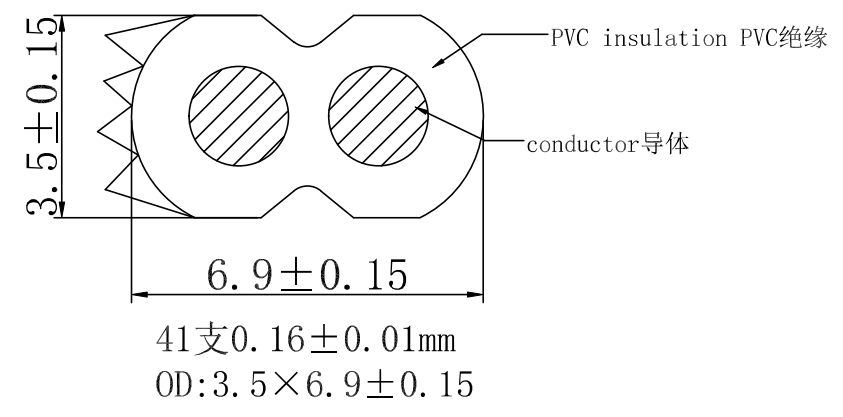
线材截面图:
