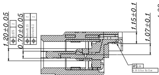
剖面图A-A
