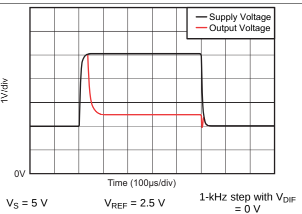
图 22. Brownout Recovery
