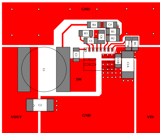
Top Layer
