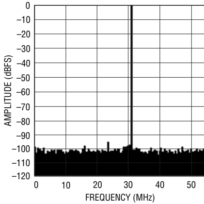
LTC2267-14: 8k Point FFT, f_{IN} = 30\text{MHz} , -1\text{dBFS} , 105\text{Mps}
