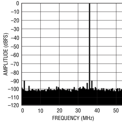
LTC2267-14: 8k Point FFT, f_{IN} = 70\text{MHz} , -1\text{dBFS} , 105\text{Mps}
