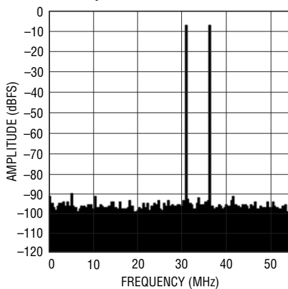
LTC2267-14: 8k Point 2-Tone FFT, f_{IN} = 70\text{MHz} , 75\text{MHz} , -1\text{dBFS} , 105\text{Mps}
