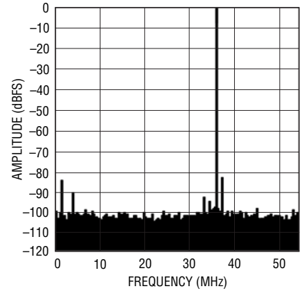
LTC2267-14: 8k Point FFT, f_{IN} = 140\text{MHz} , -1\text{dBFS} , 105\text{Mps}
