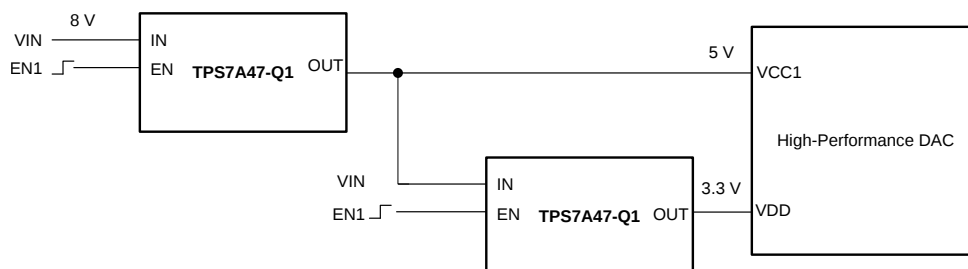
简化原理图
