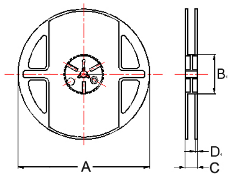
Reel Dimensions
