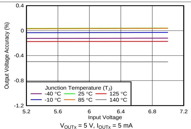
图 30. Line Regulation
