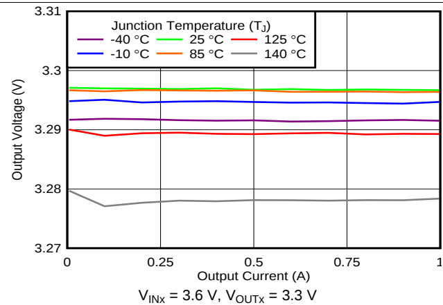
图 27. Load Regulation
