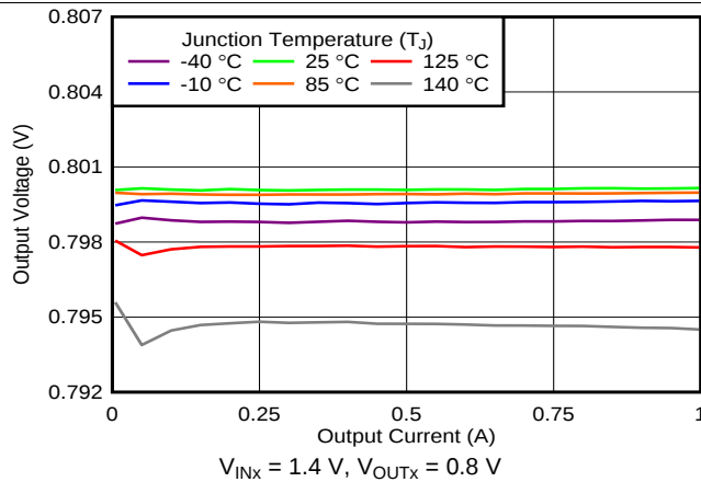
图 25. Load Regulation
