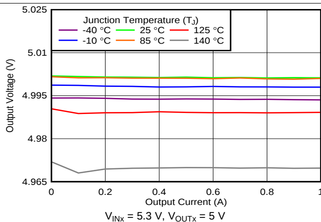
图 29. Load Regulation
