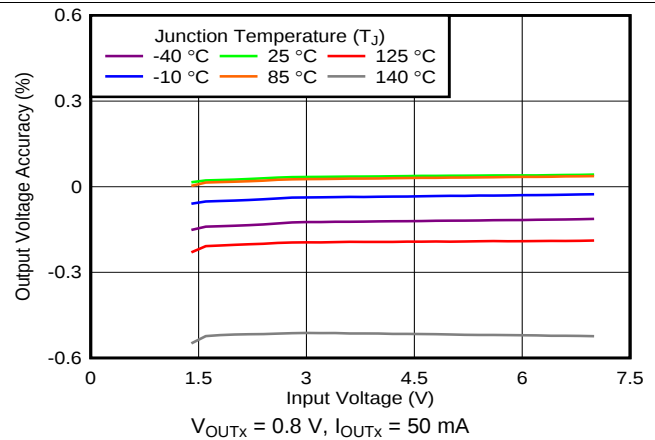
图 26. Line Regulation
