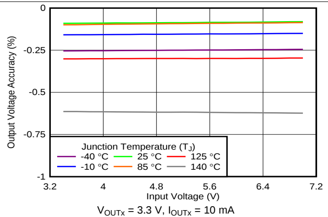
图 28. Line Regulation
