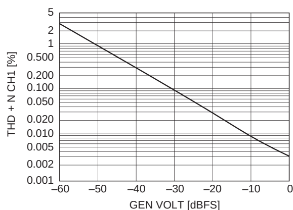
Graph 3. DAC Characteristics (C, Sch)
