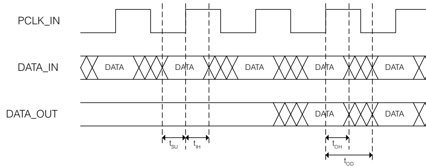
Fig. 1 Synchronous I/O Time
