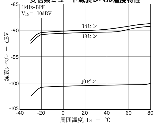
受信系ミュート減衰レベル温度特性
