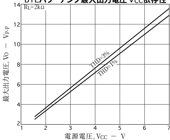
BTLパワーアンプ最大出力電圧 V_{CC} 依存性
