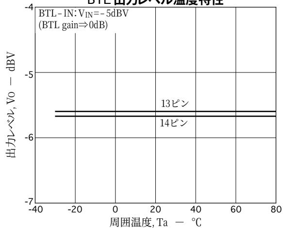
BTL 出力レベル温度特性
