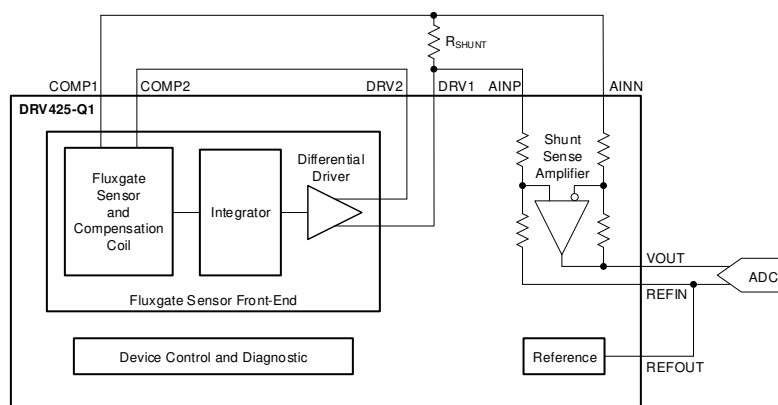
简化原理图
