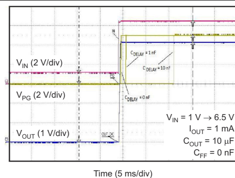
图 6-13. Power-Good Delay
