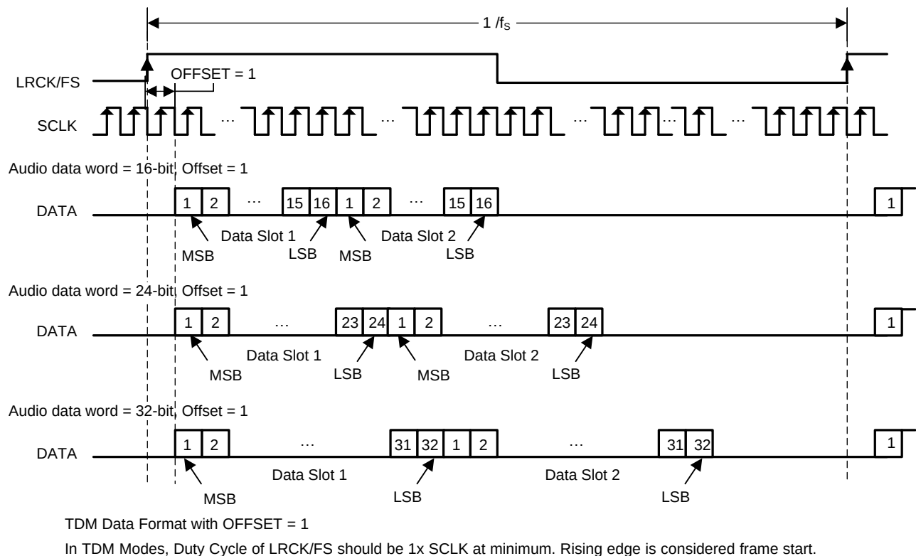
图 71. TDM 2 Audio Data Format
