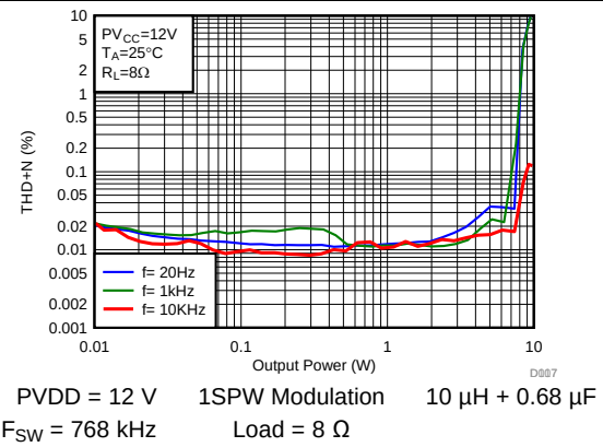
图 16. THD+N vs Output Power-BTL
