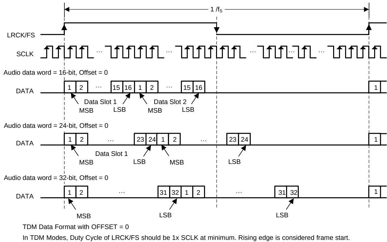
图 70. TDM 1 Audio Data Format
