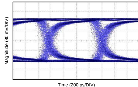
典型眼图
